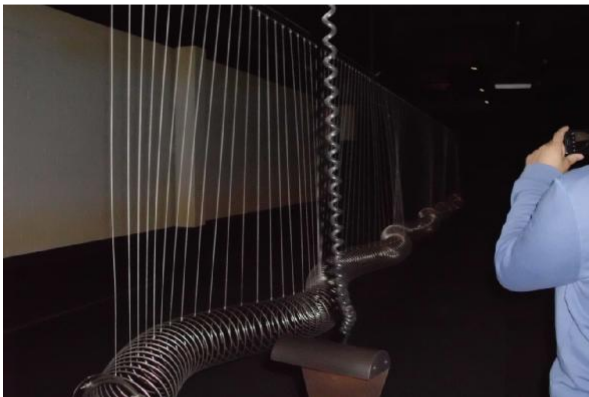
Technorama – demonštrácia vlnenia
